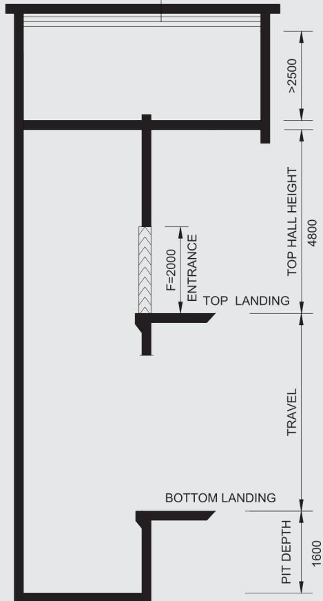
ELEVATION
